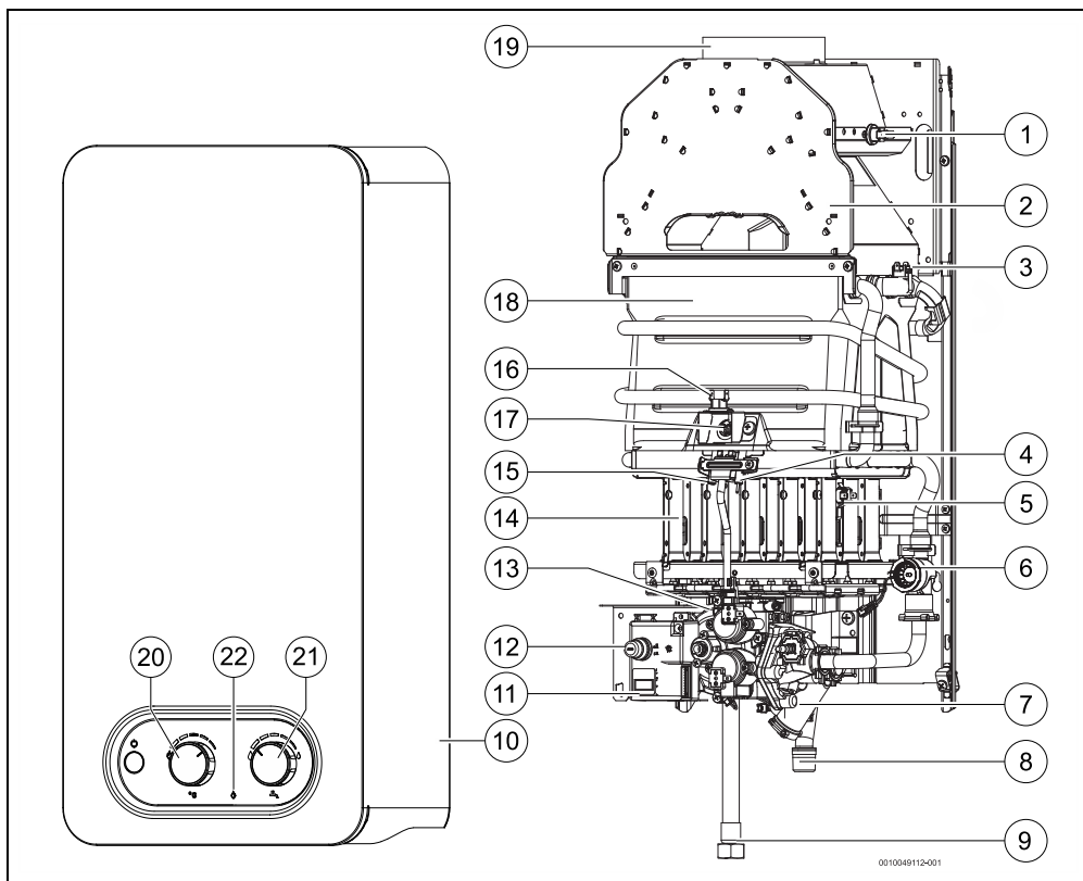
Bild 2 Gerätedesign
