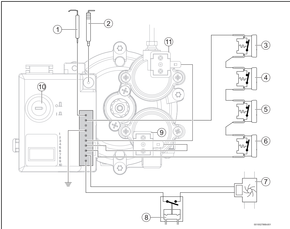
Bild 31 Schaltplan
