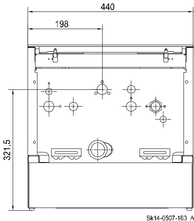
Abb. 13: Abmessung Gasanschluss bei ProCon E 20/25 mit MAG
