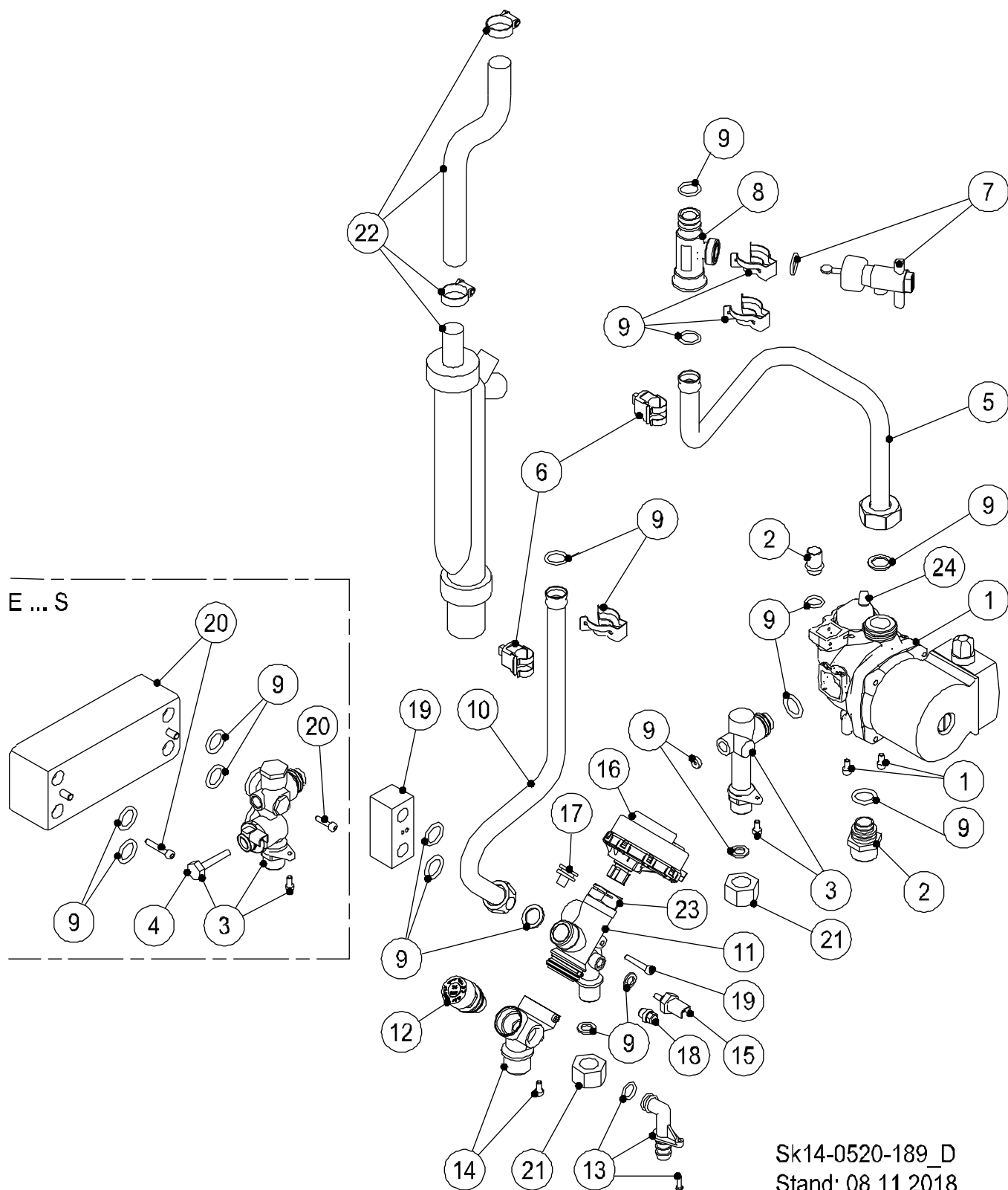
Abb. 37: Funktionsteile Hydraulik
