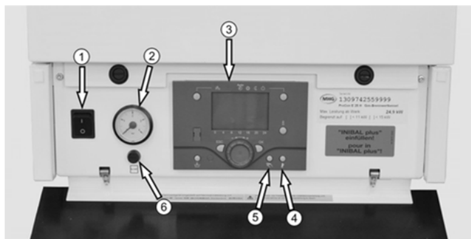
Abb. 25: Bedienkonsole
