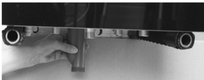
Abb. 8: Herausziehen des Siphons
