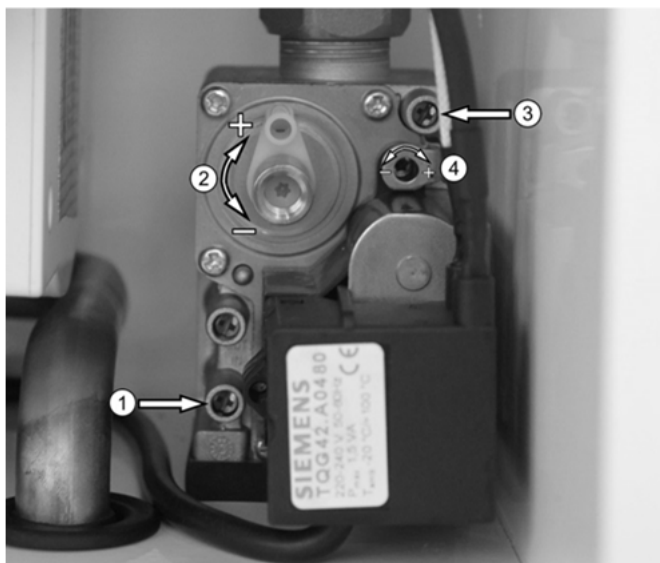
Abb. 26: Gasarmatur
