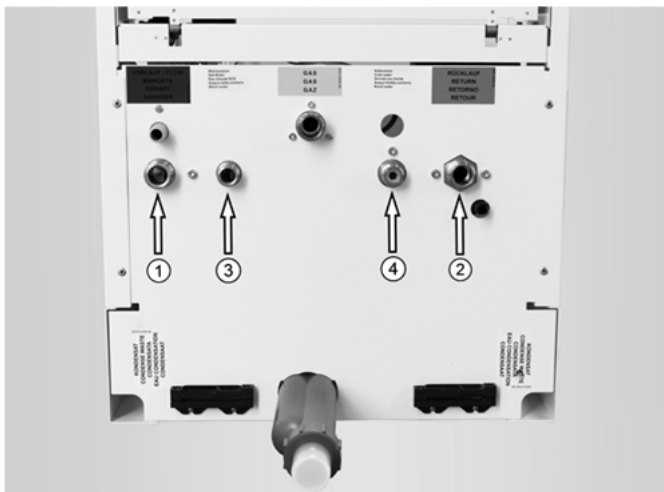
Abb. 17: Anschlusspositionen Heizungsvorlauf ① und Heizungsrücklauf ②
