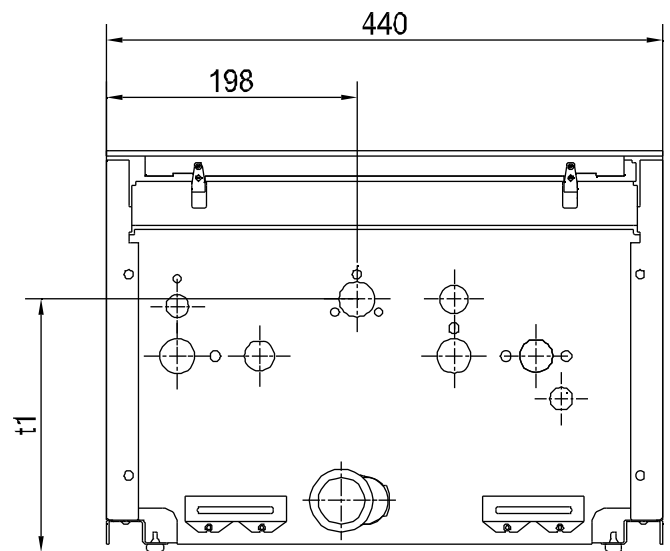
Abb. 12: Abmessung Gasanschluss
