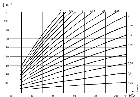
Abb. 28: Heizkennlinie (Steilheit)
