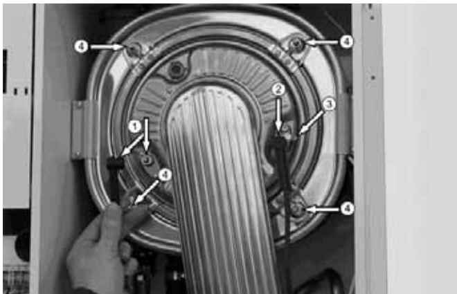
Abb. 30: Brenner und Brennerplatte
