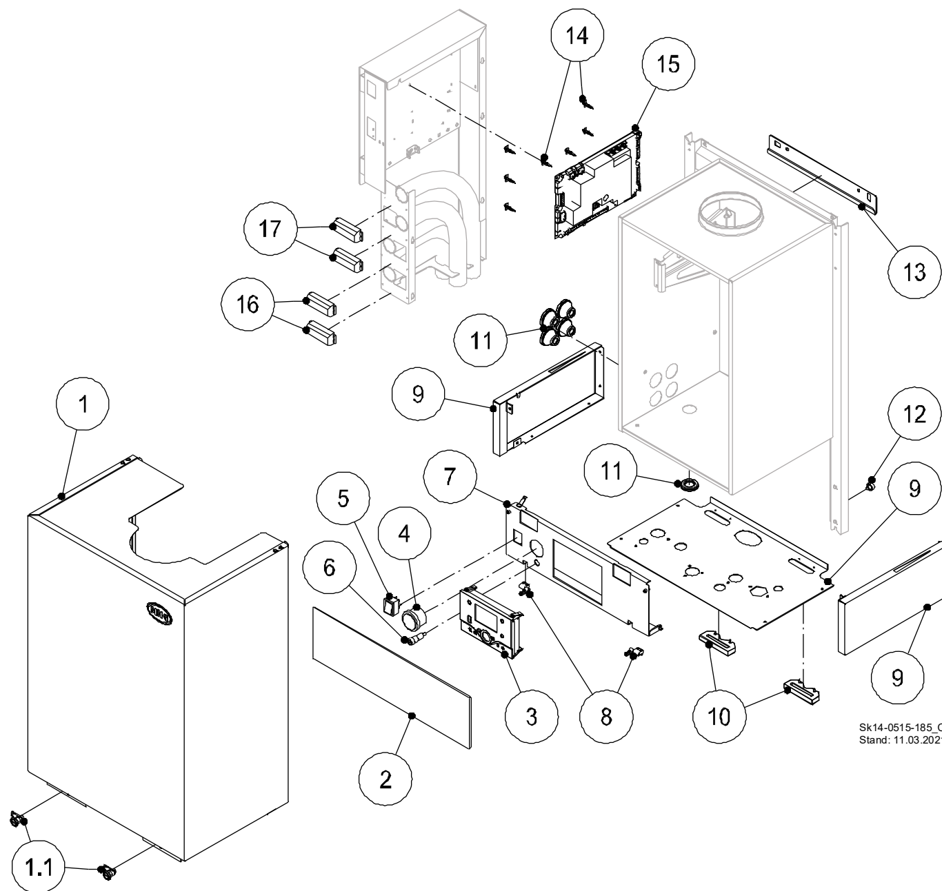
Abb. 36: Gehäuseteile und Regelung
