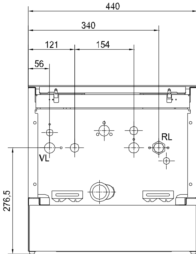
Abb. 16: Abmessungen Heizungsvorlauf (VL) und Heizungsrücklauf (RL) bei ProCon E 20/25 mit MAG
