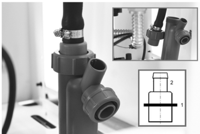
Abb. 9: Montage Schlauchanschluss
