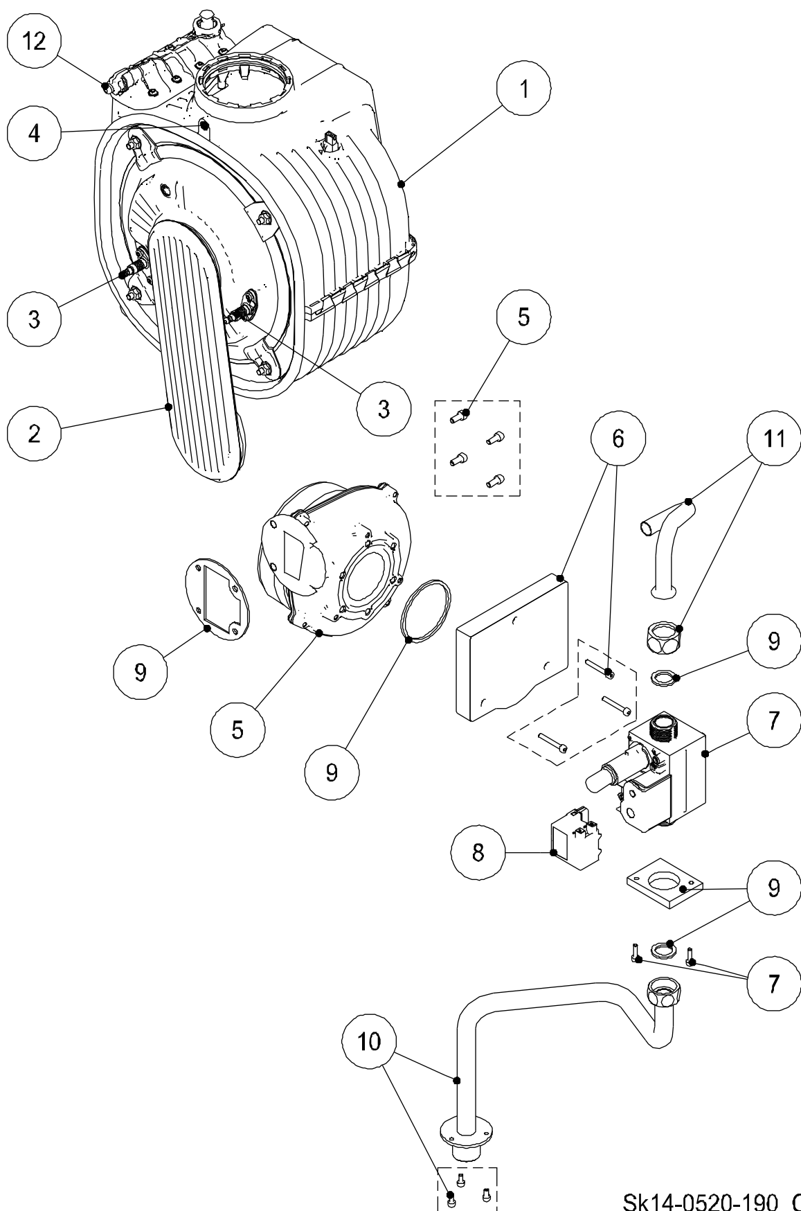
Abb. 38: Kesselkörper
