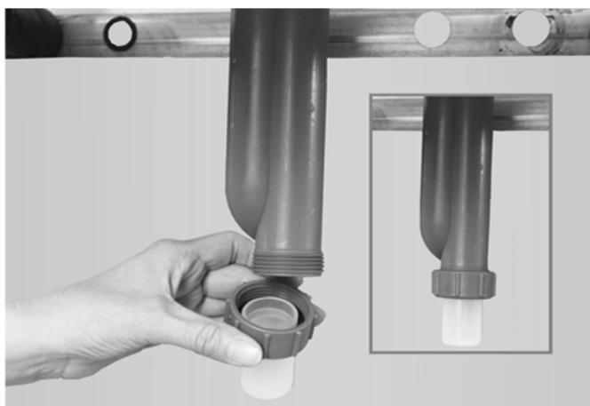
Abb. 10: Montage Schmutzkorb
