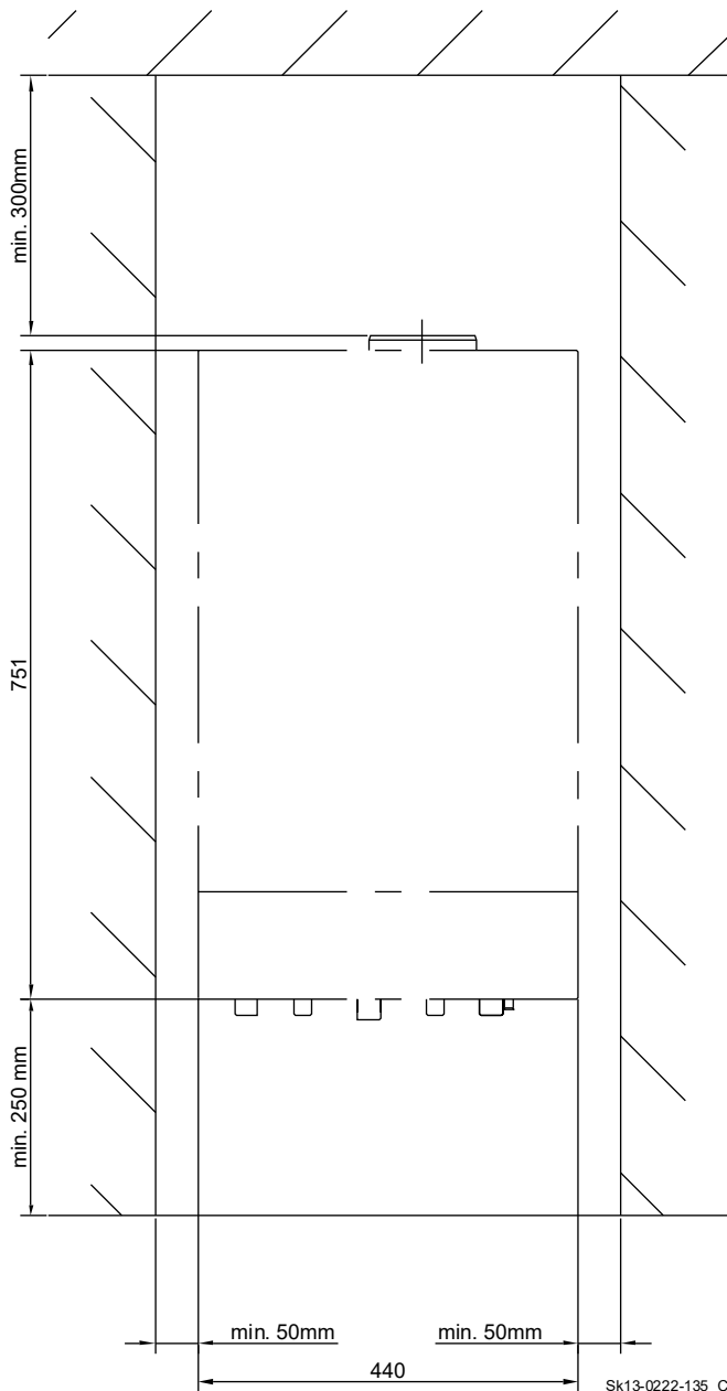
Abb. 1: Montageabstände
