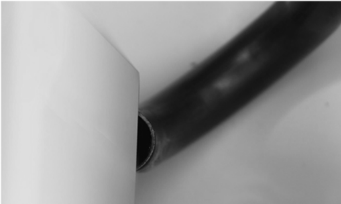
Abb. 33: Falsche Einbauposition des Gasrohres am Gas-Luft-Mischkasten
