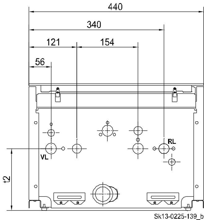
Abb. 15: Abmessungen Heizungsanlauf (VL) und Heizungsrücklauf (RL)
