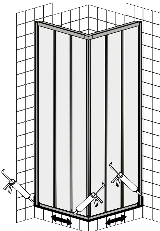
Eckeinstieg 4- und 6-teilig 4 and 6-part corner entry
