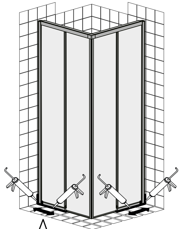
Eckeinstieg 4-teilig barrierefrei 4-part corner entry barrier-free
