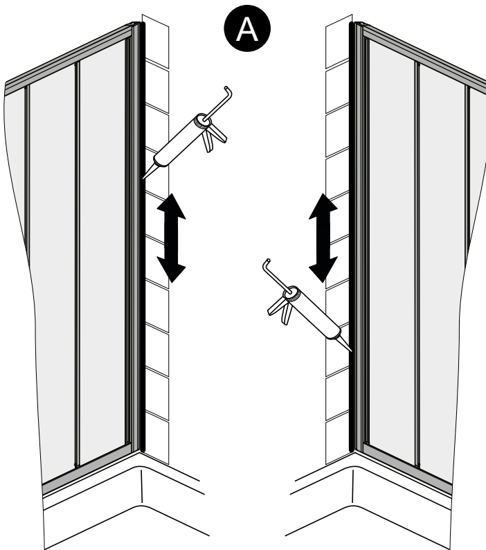
Eckeinstieg 4-teilig barrierefrei 4-part corner entry barrier-free
